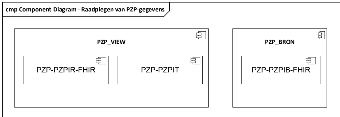
Figuur 7: Component Diagram voor Raadplegen van PZP-gegevens
